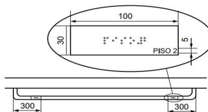
b) Sinalização de corrimão – Vista superior
