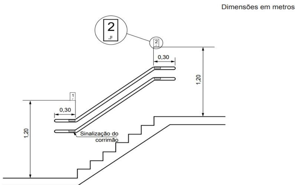
a) Sinalização de pavimento – Vista lateral
